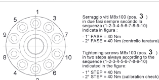
SERRAGGIO VITI SUPPORTO GUARNIZIONI TIGHTENING GASKET SUPPORT SCREWS
