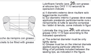
LUBRIFICAZIONE ANELLO DI TENUTA SEAL RING LUBRICATION
